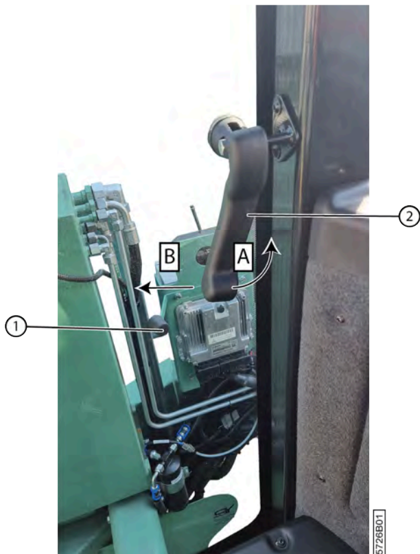
Fig. 51: Sortie de secours
