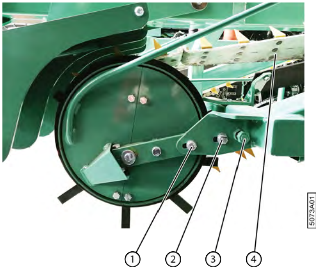
Fig. 112: Régler la tension des courroies
