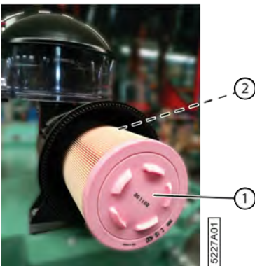
Fig. 162: Élément principal et élément de sécurité du filtre à air
