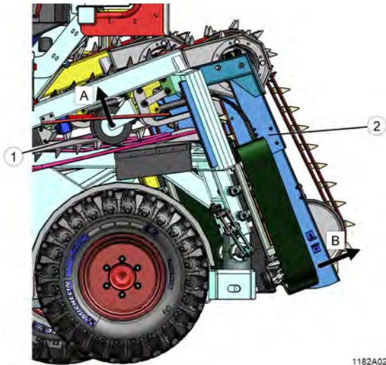
Fig. 92: Retirer un bourrage
