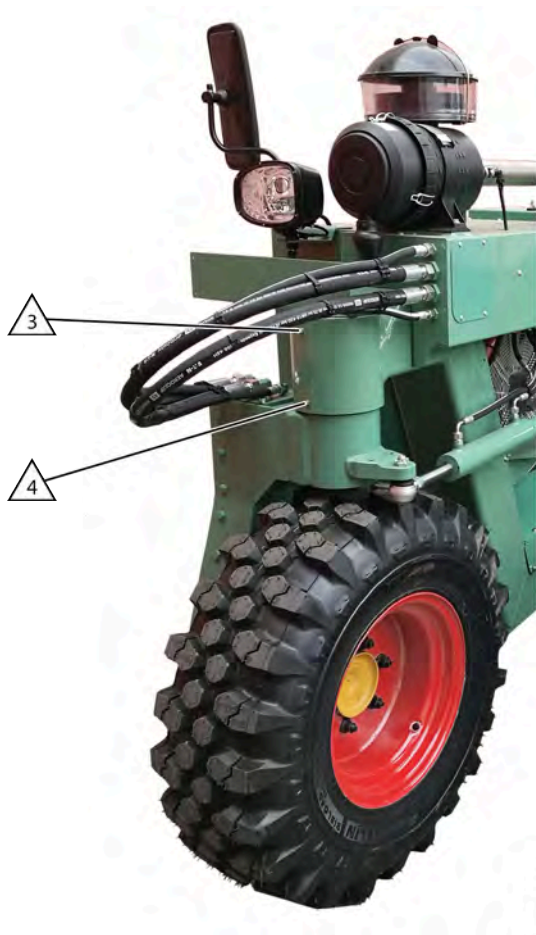
Fig. 138: Lubrifier la roue avant
