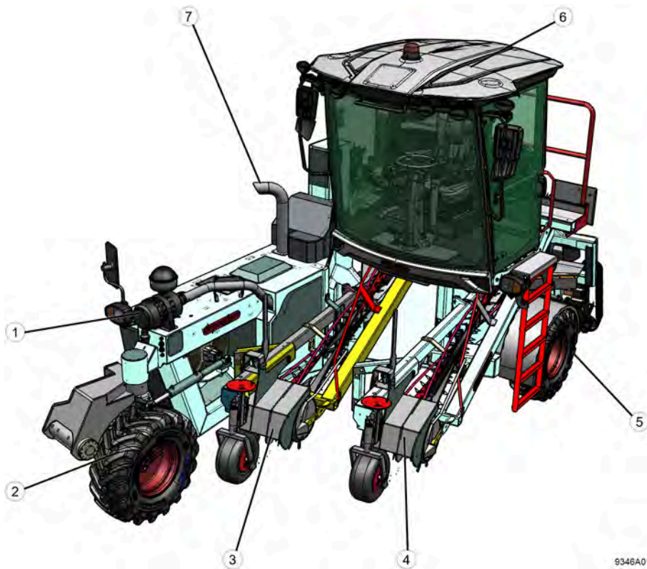
Fig. 8: Vue de face de la machine
