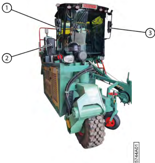
Fig. 13: Emplacement des rétroviseurs
