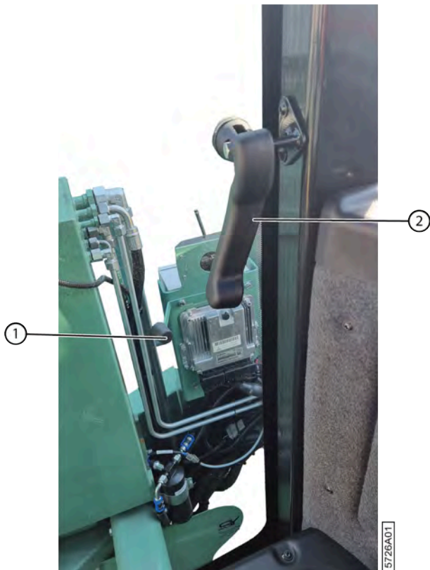
Fig. 12: Porte d'urgence
