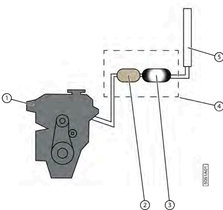
Fig. 153: Système de post-traitement des gaz d'échappement
