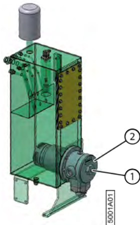
Fig. 122: Filtre d'aspiration réservoir hydraulique
