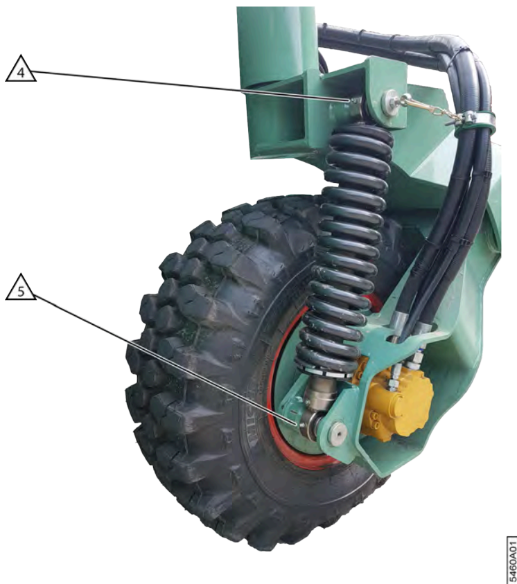
Fig. 140: Lubrifier la suspension de la roue avant
