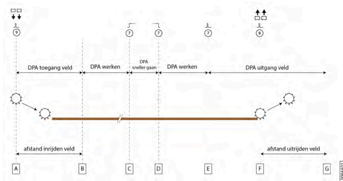
Fig. 95: DPA et distance pendant le rodage et l'épandage
