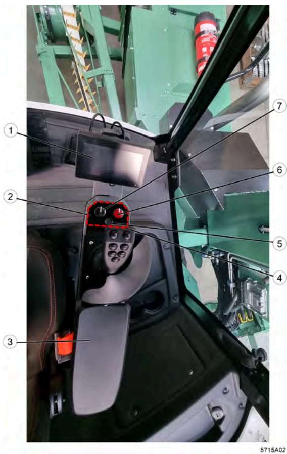
Fig. 26: Unité de commande
