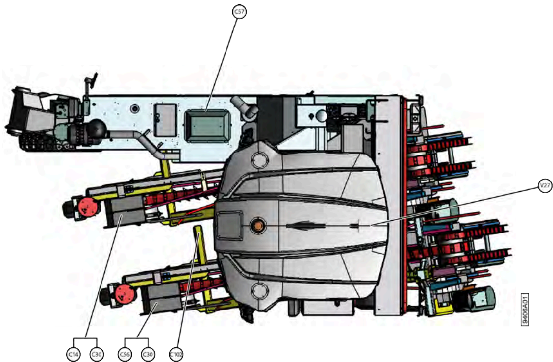
Fig. 56: Vue de dessus
