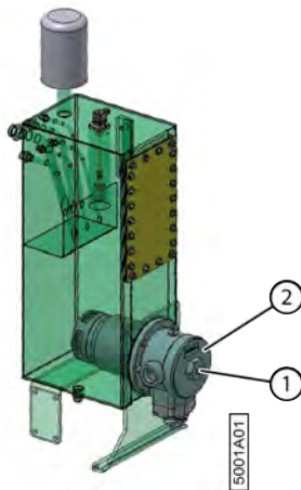
Fig. 131: Filtre d'aspiration réservoir hydraulique
