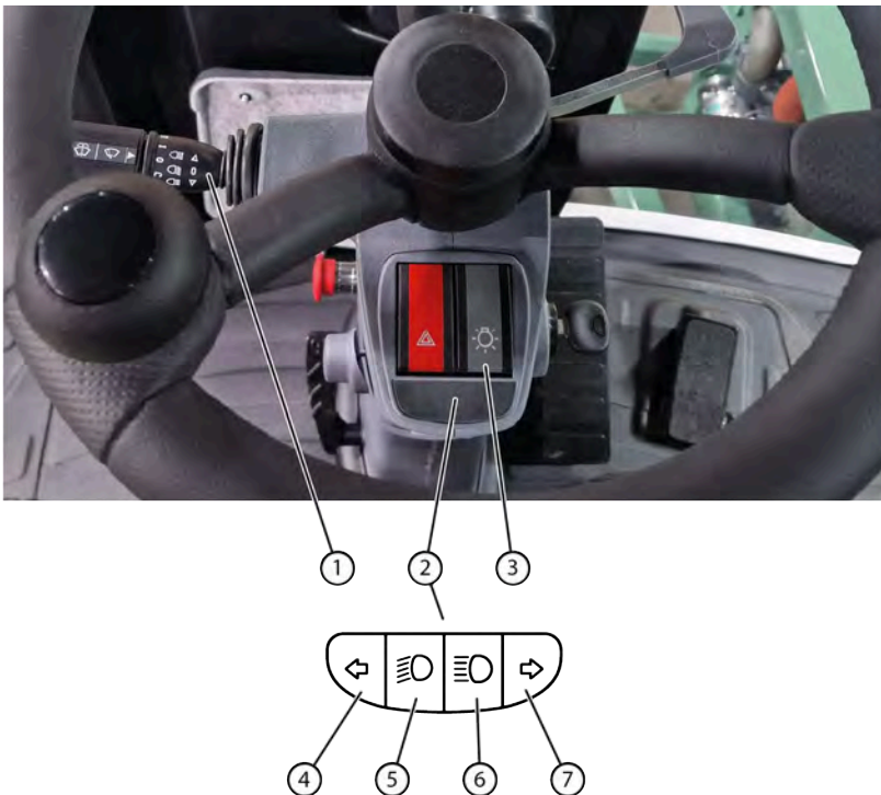
Fig. 73: Boutons sur le volant
