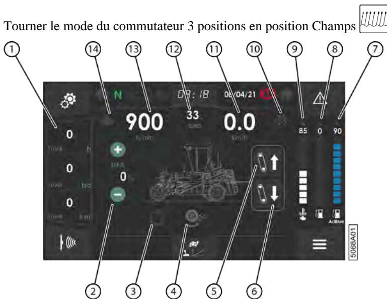
Fig. 81: Fenêtre du mode Champs
