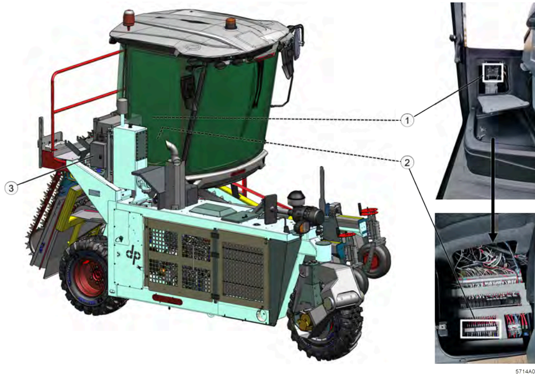
Fig. 152: Emplacement des fusibles
