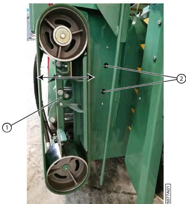
Fig. 119: Régler la courroie d'alignement côté pied
