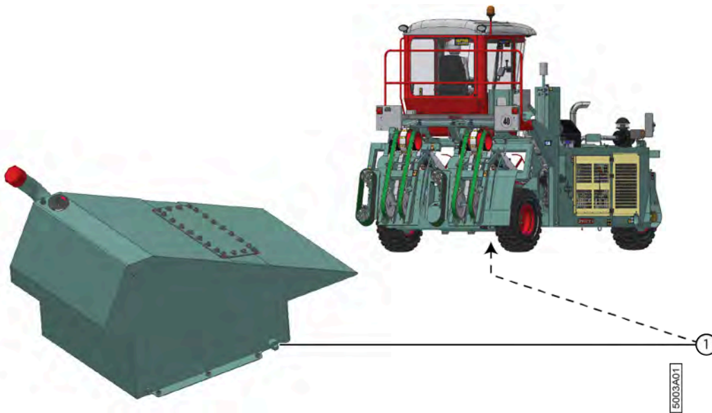
Fig. 158: Vidanger le réservoir à carburant
