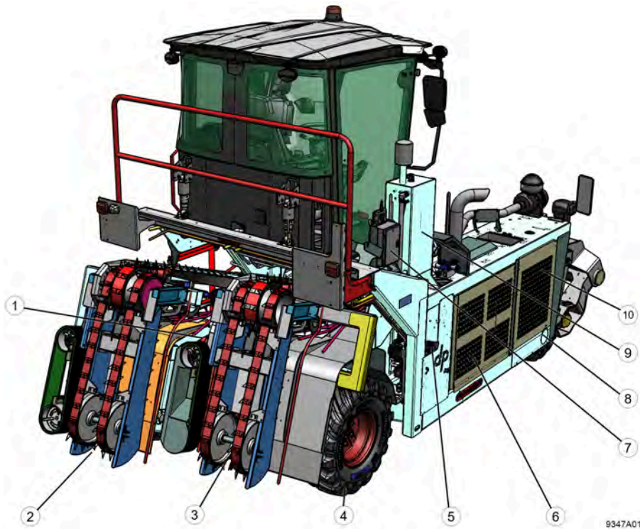
Fig. 9: Vue arrière
