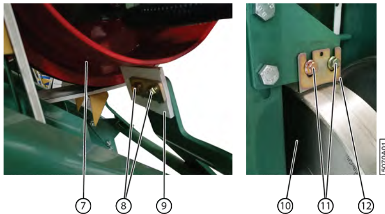
Fig. 115: Régler les racleurs
