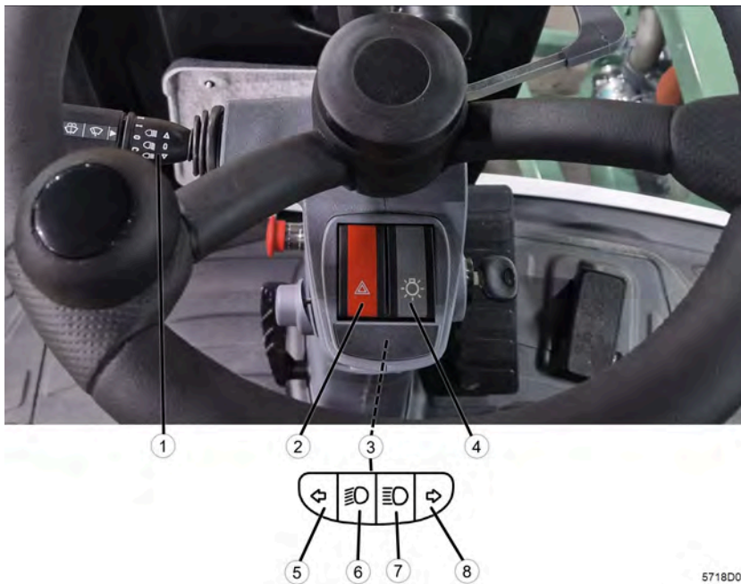
Fig. 20: Boutons sur le volant
