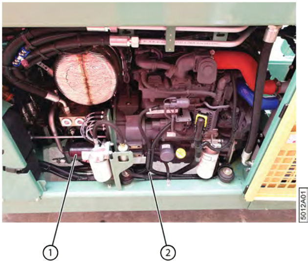
Fig. 121: Remplacer les filtres de pression de gavage
