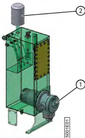
Fig. 166: Filtres sur le réservoir hydraulique
