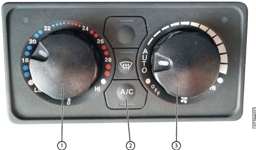
Fig. 102: Mettre l'air conditionné en mode automatique
