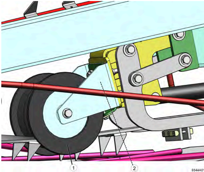
Fig. 118: Régler le galet de roulement d'une courroie de transport
