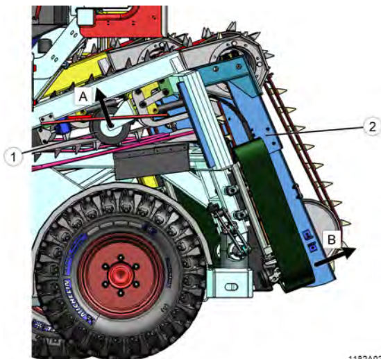
Fig. 91: Retirer un bourrage
