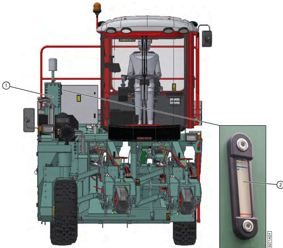
Fig. 128: Niveau huile hydraulique
