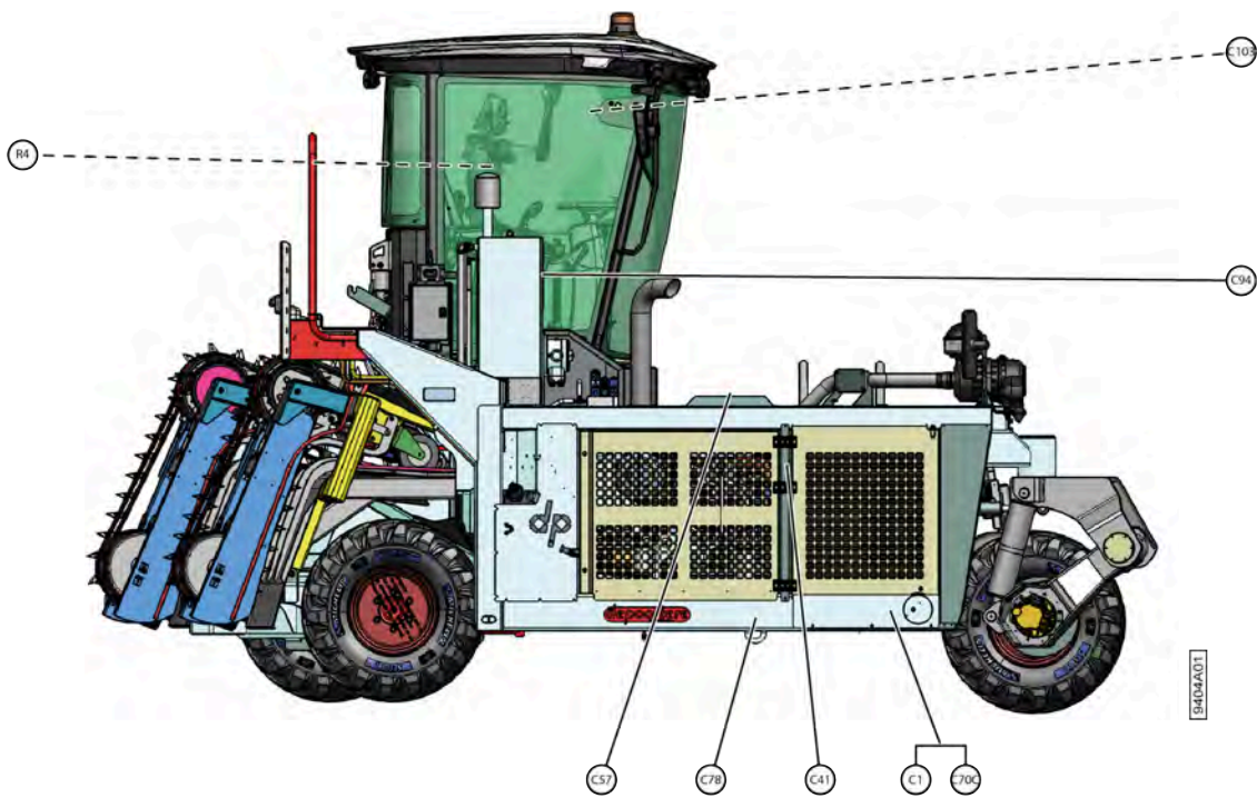
Fig. 54: Vue de droite
