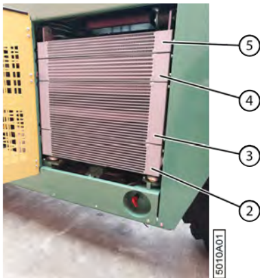
Fig. 124: Nettoyer les radiateurs
