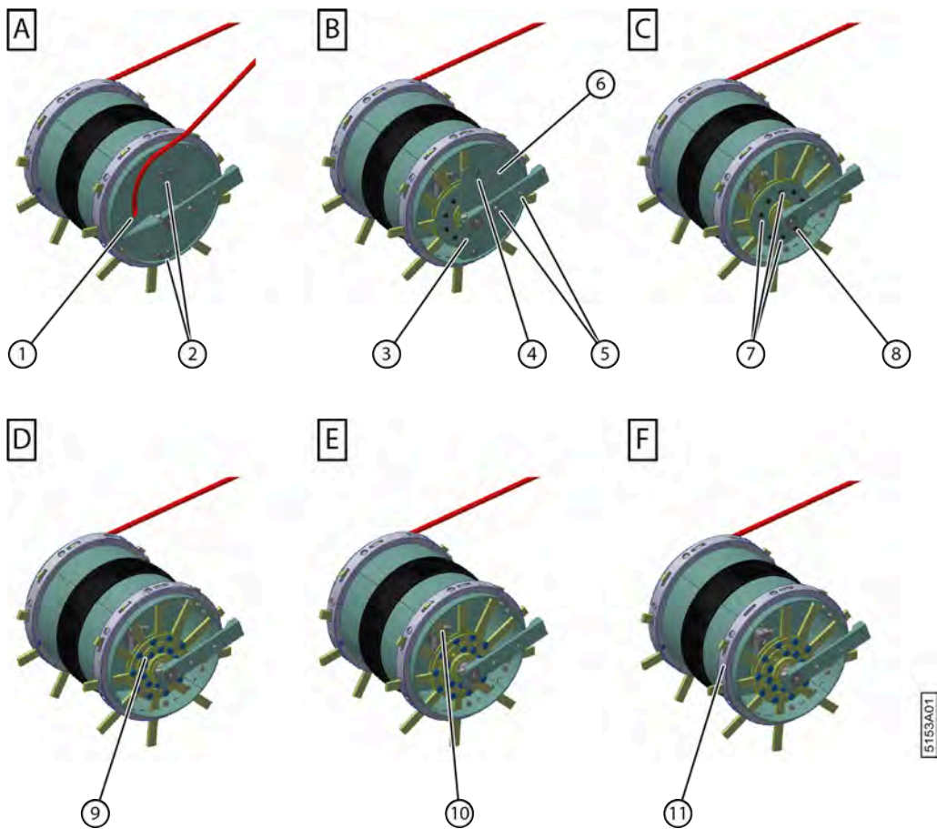
Fig. 149: Remplacer la dent du tambour de pick-up
