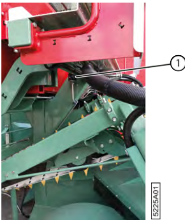
Fig. 136: Filtre d'aération du réservoir à carburant
