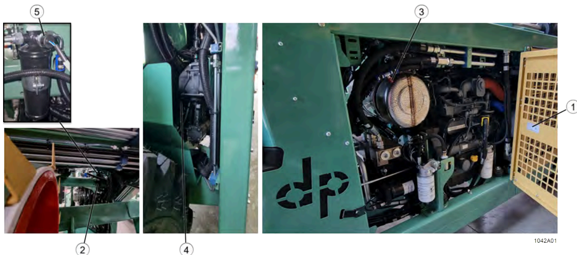
Fig. 132: Position des éléments de l'air conditionné
