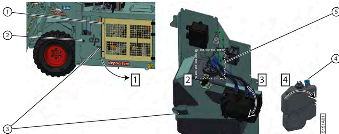
Fig. 61: Démontez et vidanger le réservoir d'AdBlue
