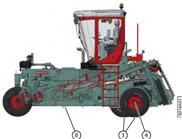
Fig. 145: Anneau de remorquage de la machine
