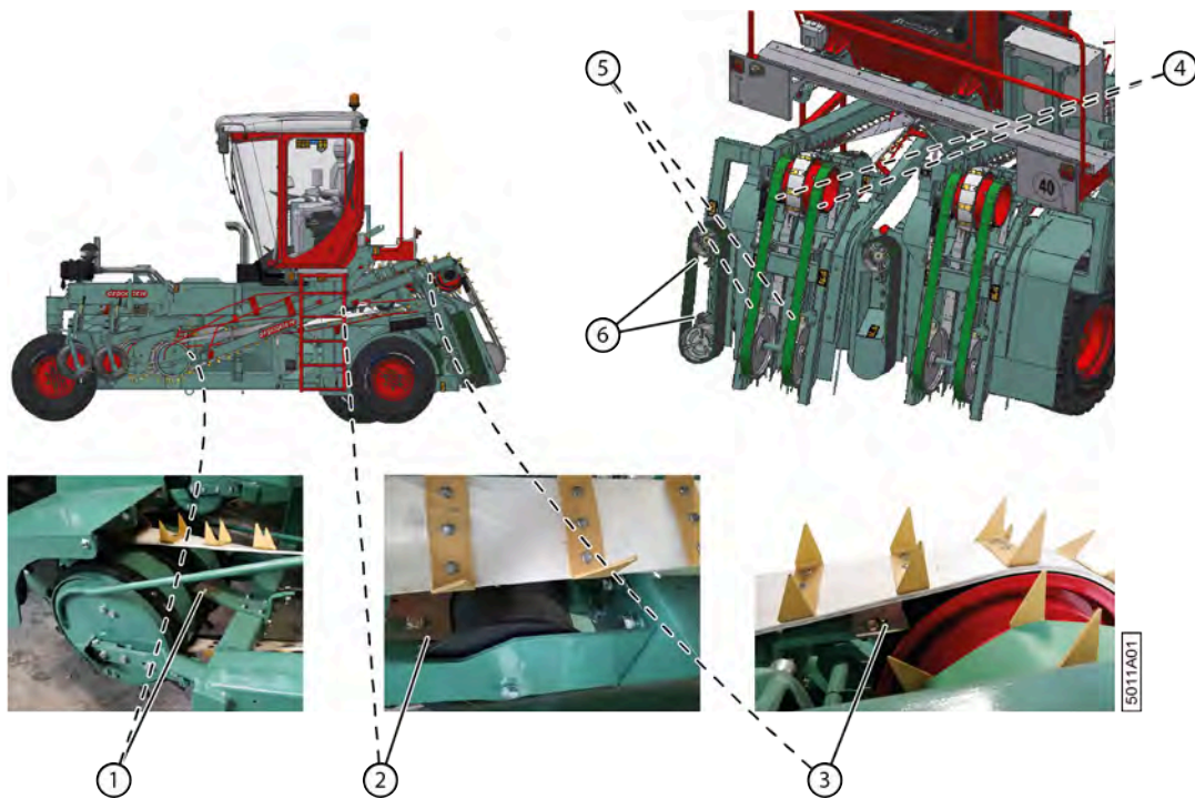
Fig. 114: Emplacement des racleurs
