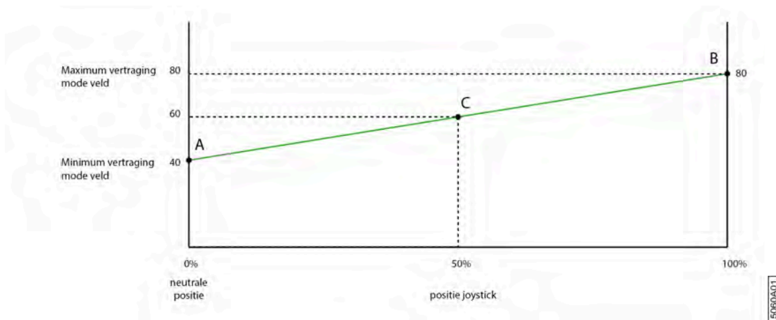
Fig. 96: Exemple de ralentissement en mode champs alors que la vitesse de réaction est réglée sur variable
