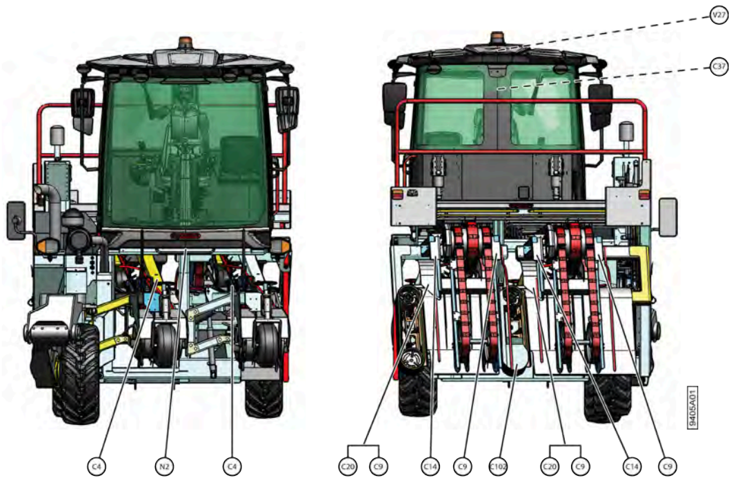
Fig. 53: Vue avant et vue arrière
