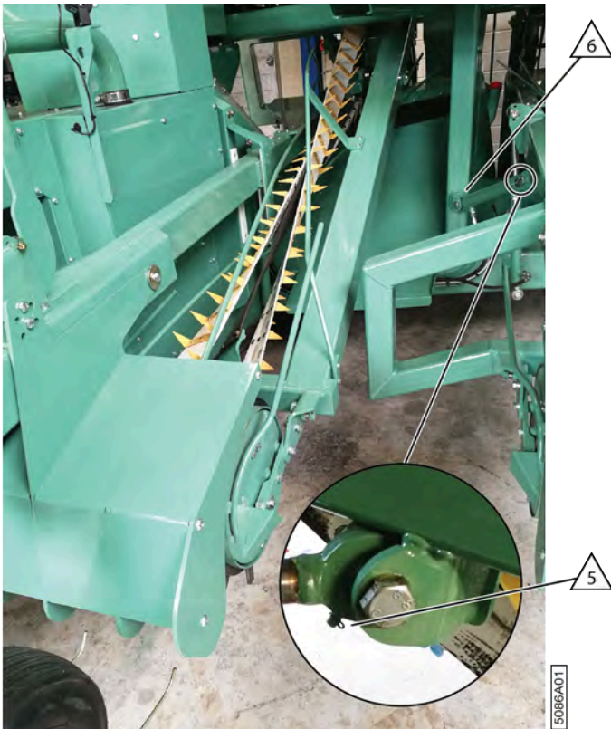
Fig. 139: Lubrifier le vérin du pick-up gauche
