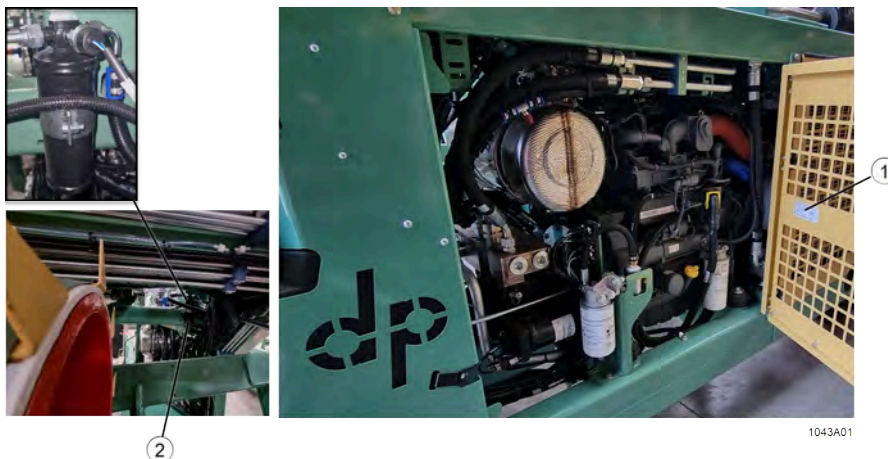
Fig. 134: Position du filtre à sec de l'air conditionné
