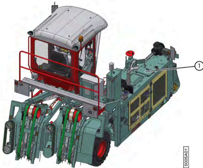
Fig. 46: Emplacement de la boîte à outils
