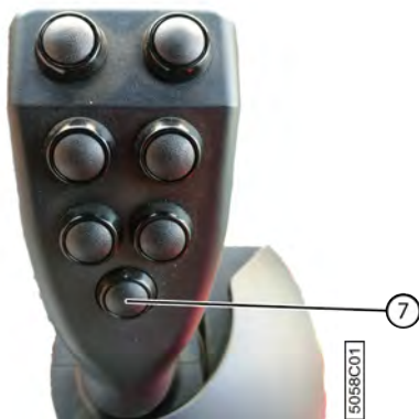
Fig. 89: Activer/désactiver le mode sortie avec le joystick
