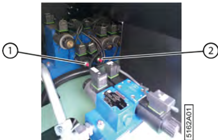
Fig. 97: Commande manuelle
