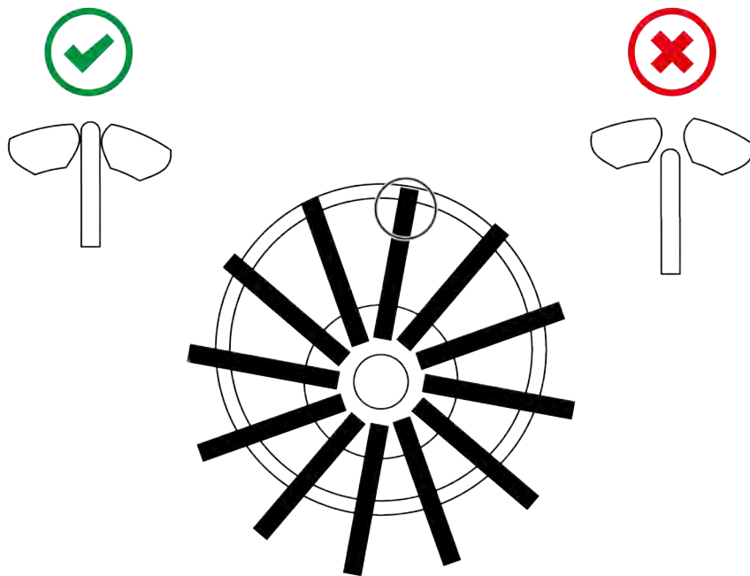
Fig. 125: Les dents du pick-up
