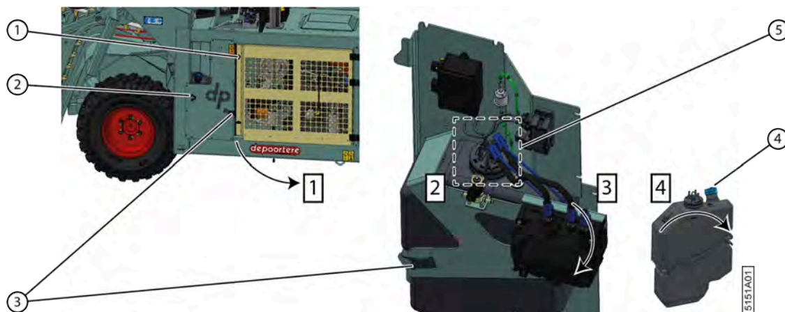
Fig. 159: Démontez et vidanger le réservoir d'AdBlue
