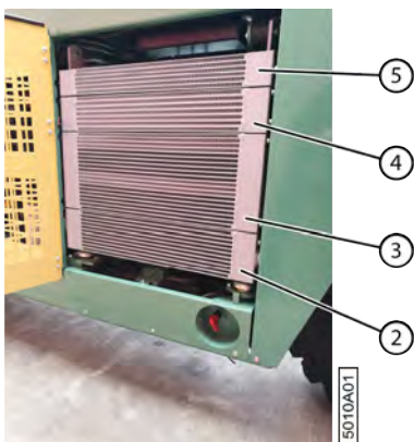
Fig. 45: Radiateurs
