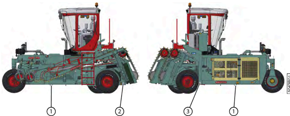
Fig. 58: Fixer la machine sur le camion
