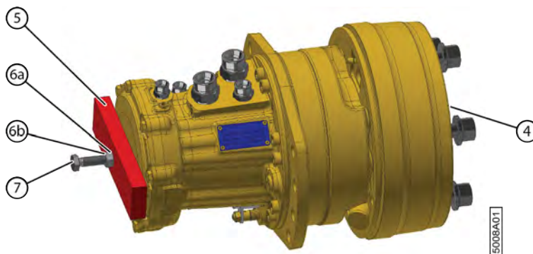
Fig. 144: Ouverture du frein
