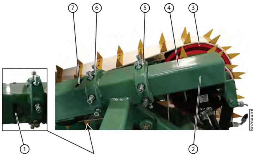
Fig. 117: Régler la roue motrice
