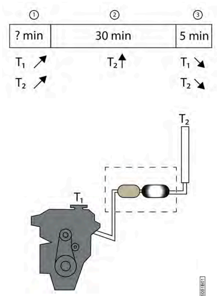
Fig. 154: Les 3 phases d'une régénération après arrêt
