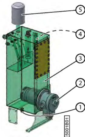
Fig. 40: Réservoir hydraulique
