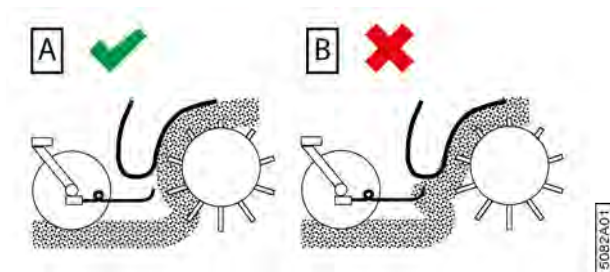
Fig. 110: Réglages possibles des tiges de guidage en forme de queue de cochon de la roue de jauge
