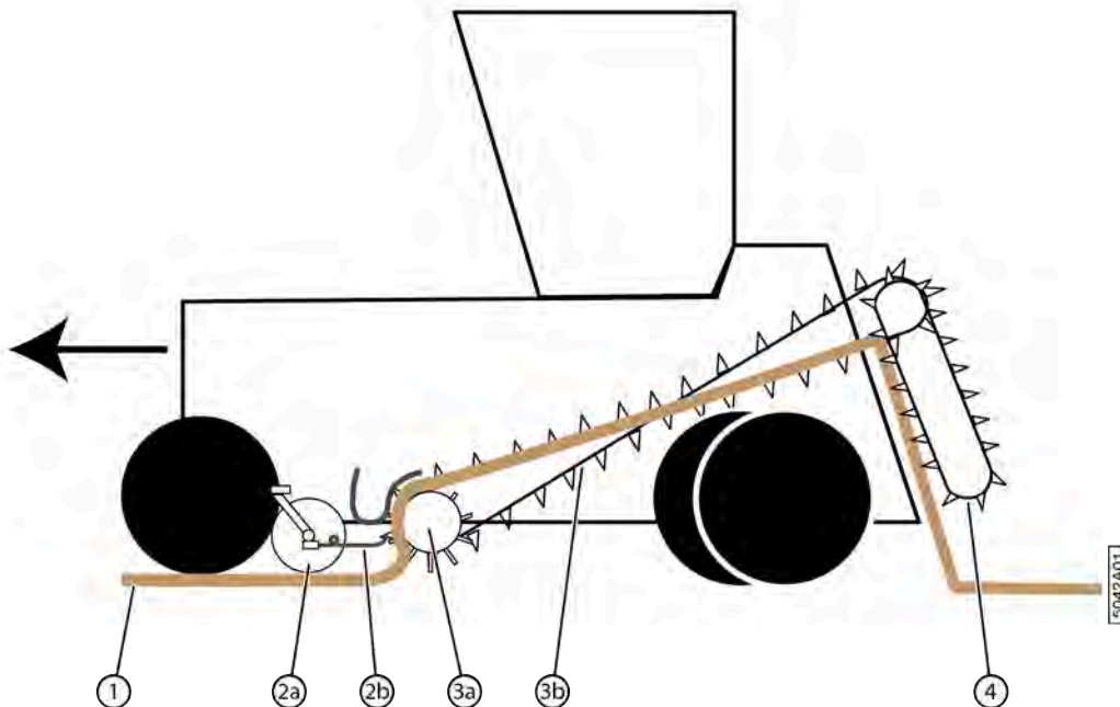
Fig. 47: Fonctionnement de la double retourneuse automotrice hydraulique
