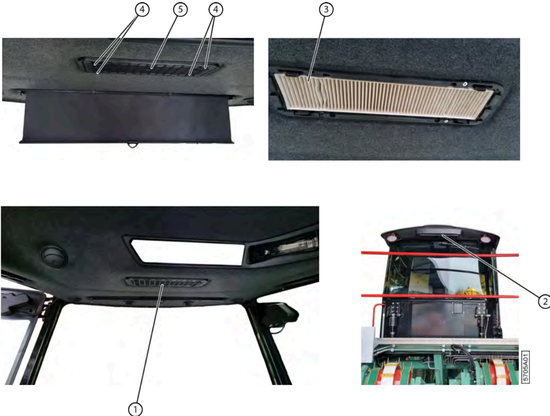
Fig. 127: Filtrés à air de la cabine
