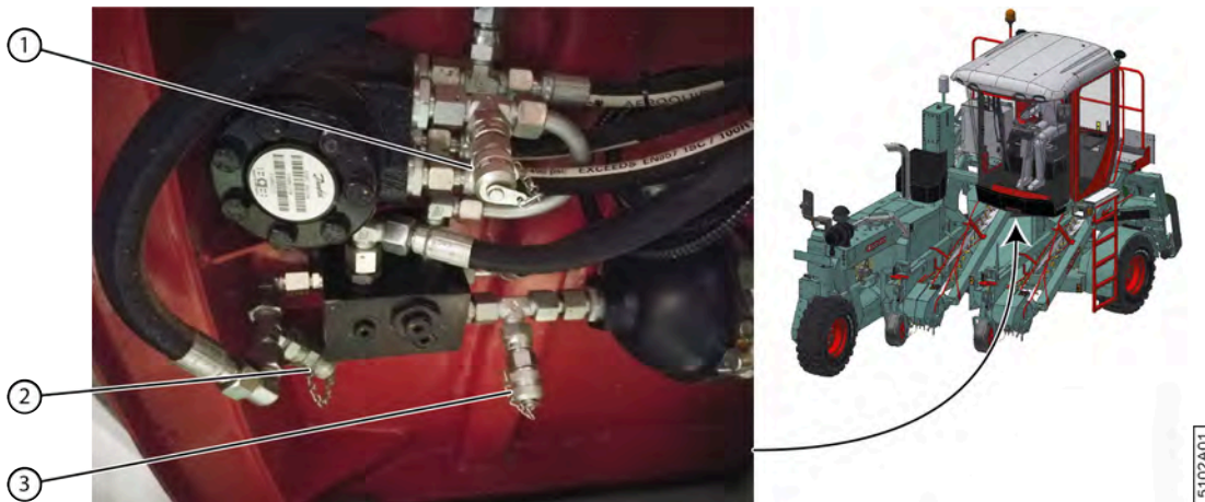
Fig. 155: Sous la cabine
