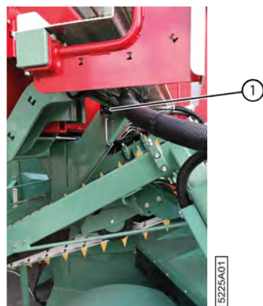
Fig. 164: Filtre d'aération du réservoir à carburant
