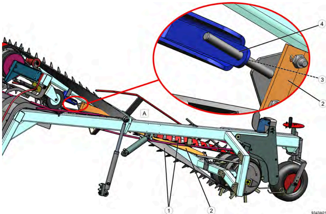
Fig. 116: Régler la tension de la courroie intermédiaire
