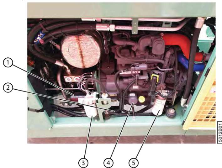
Fig. 163: Filtres dans le compartiment moteur
