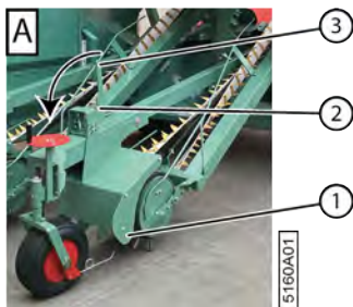
Fig. 94: Ouvrir le contre pick-up
