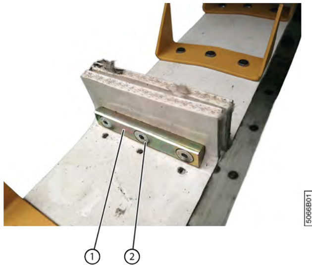
Fig. 148: Remplacer une courroie de transport
